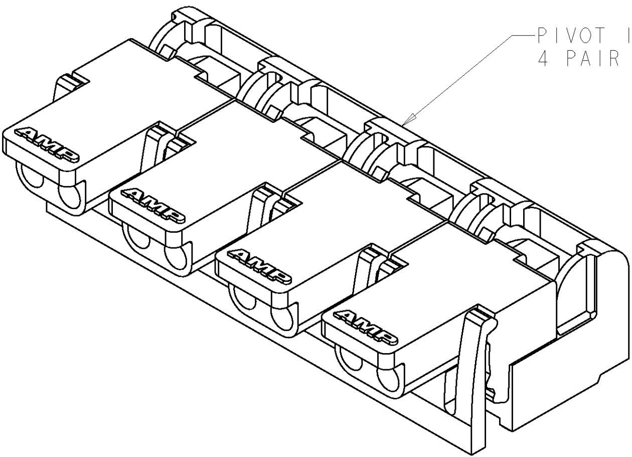
1339376-2 SHOWN SCALE 4:1
