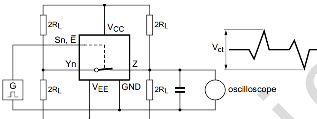
图14、测量控制输入与任何开关之间的串扰测试线路
