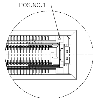
DETAIL E (SCALE 4:1)
