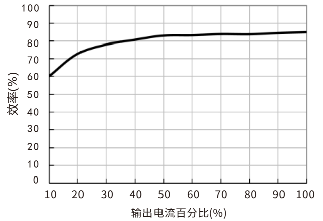
效率Vs输出负载(Vin=12V)
