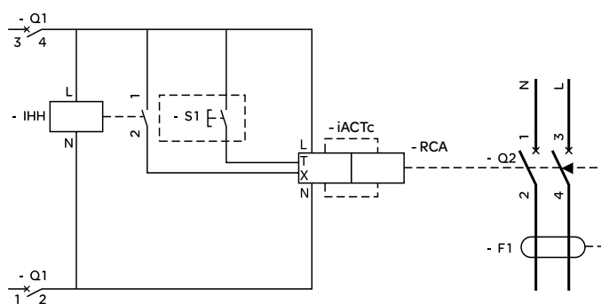
控制回路
