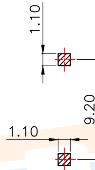
PCB Layout(Pattern Side)
