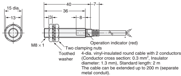
Diagram 5 E2E-X3D□ E2E-X2E□/F□
