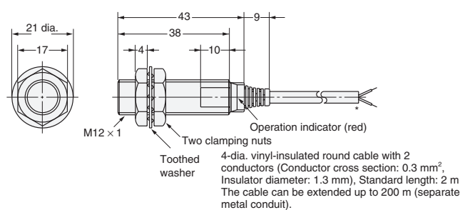
Diagram 7 E2E-X2Y□
