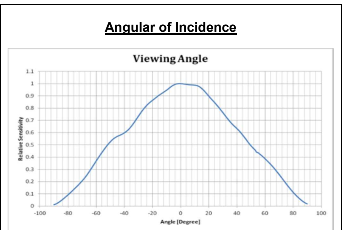
Figure 4.2 ALS Sensitivity vs. Angular of Incidence
