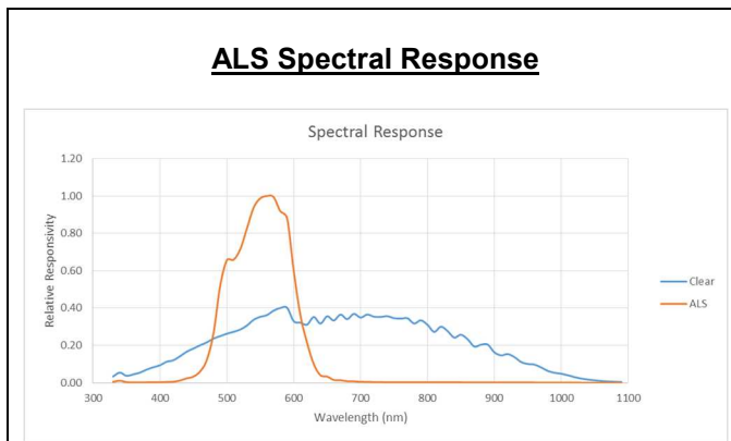
Figure 4.1 Spectral Response of ALS & CLEAR Channels
