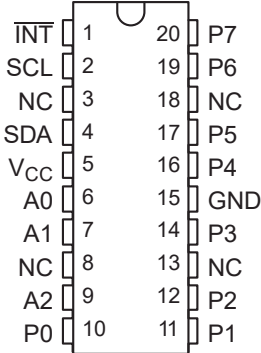
TSSOP20
