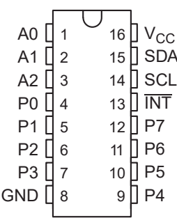
SOP16
