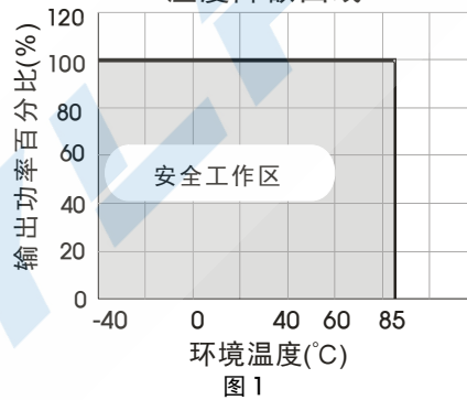
温度降额曲线
