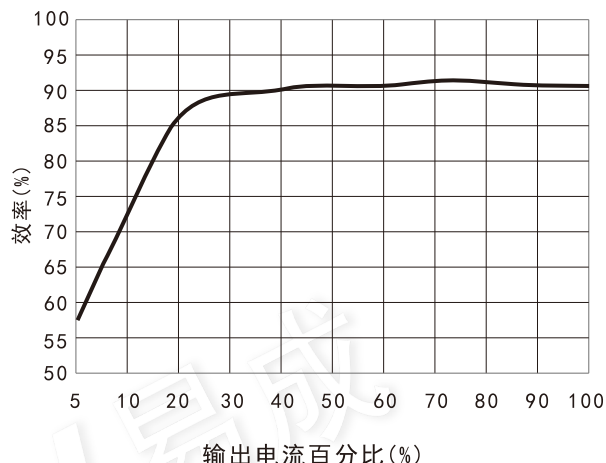
效率Vs输出负载 (Vin=48V) VRB4815LD-15WR3
