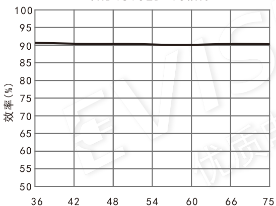
效率Vs输入电压(满载) VRB4815LD-15WR3
