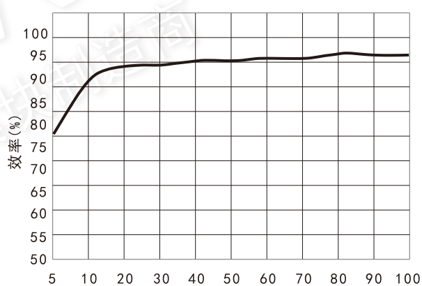
效率Vs输出负载 (Vin=48V) VRB4815LD-15WR3
